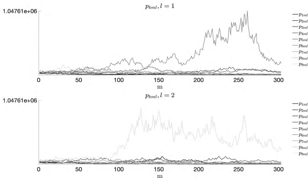
Рис. 3. Визуализация изменения цен на всем горизонте планирования.
