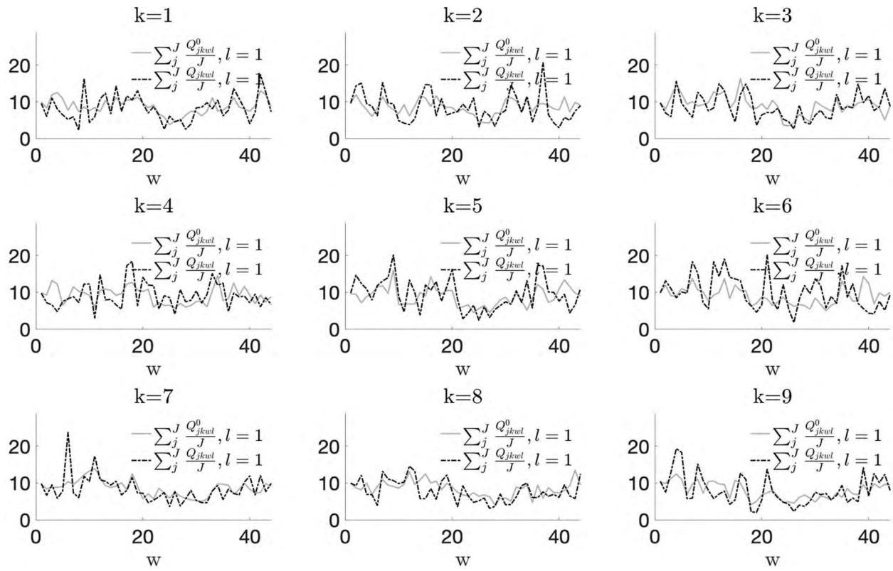
Рис. 4. Визуализация исходного и текущего спроса с учетом изменений при поиске вектора цен для l = 1 .
