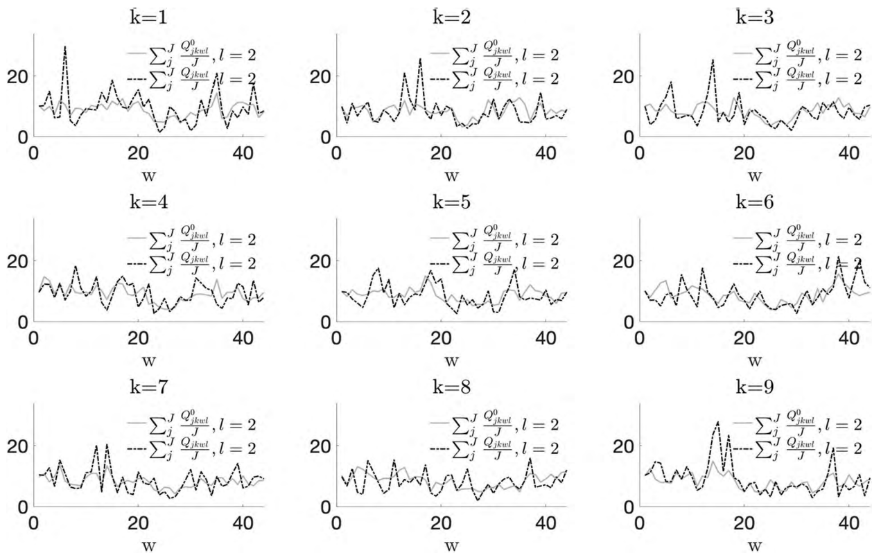
Рис. 5. Визуализация исходного и текущего спроса с учетом изменений при поиске вектора цен для l = 2 .
