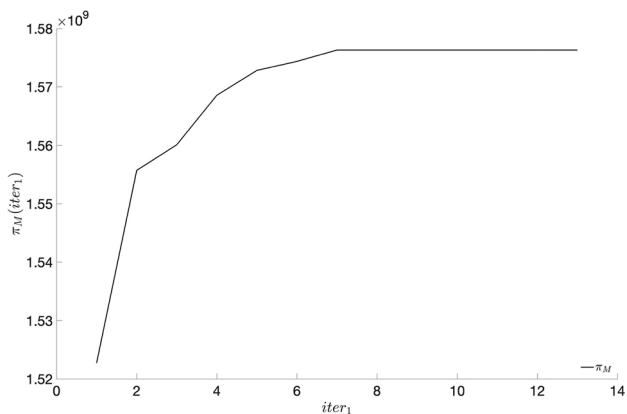
Рис. 1. Визуализация значений накопленной прибыли в зависимости от номера итерации iter_1 .
