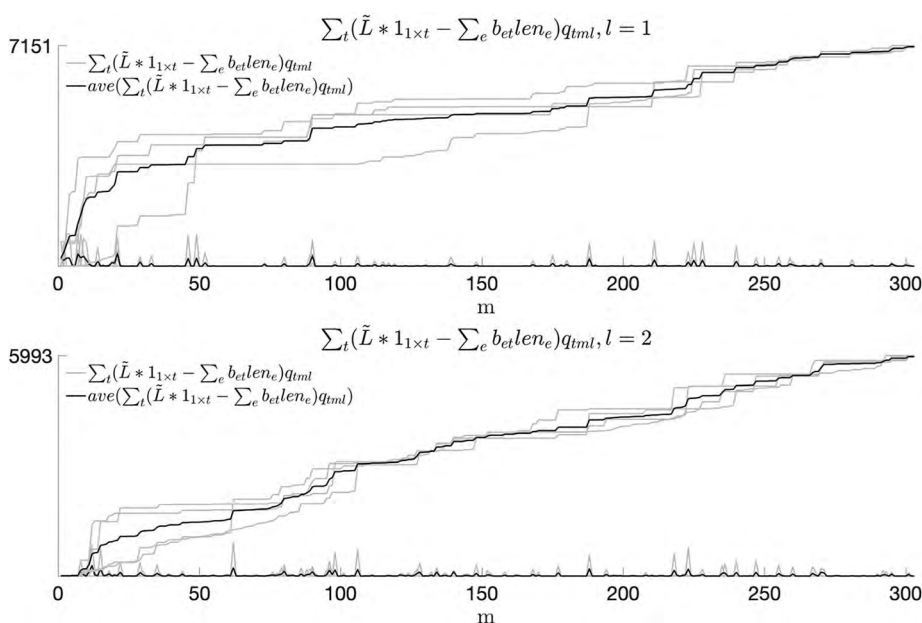
Рис. 6. Визуализация объемов суммарных отходов сырья.
