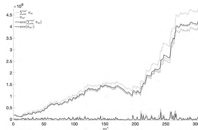
Рис. 2. Визуализация тестирования полученного решения.
