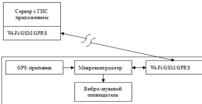
Рисунок 1. Логическая схема работы устройства
