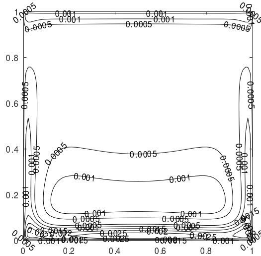
Рис. 1. Относительная разница между полями температуры в моделях P_1 и SP_3 .
