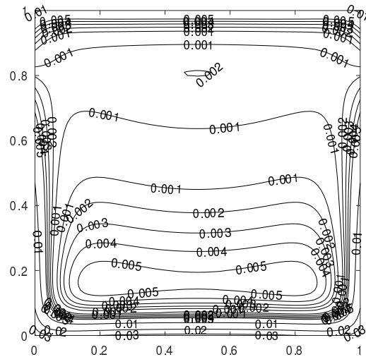
Рис. 2. Относительная разница между полями интенсивности излучения в моделях P_1 и SP_3 .
